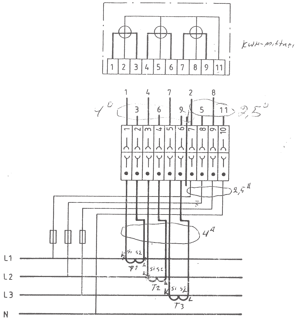
Kuva 2 Epäsuora mittaus, virtamuuntajaliitäntä (SFS 2537 kytkentä 4010)
